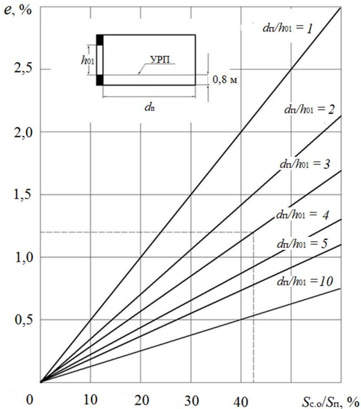
Рисунок 6.8 – График для определения КЕО e_{cp} при боковом освещении помещений производственных зданий и рабочих кабинетов
